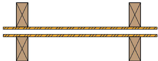
Mur 8: double ossature, voile travaillant côté lame d'air
