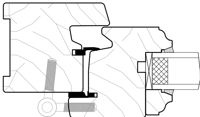
double joint central sur dormant et recouvrement
