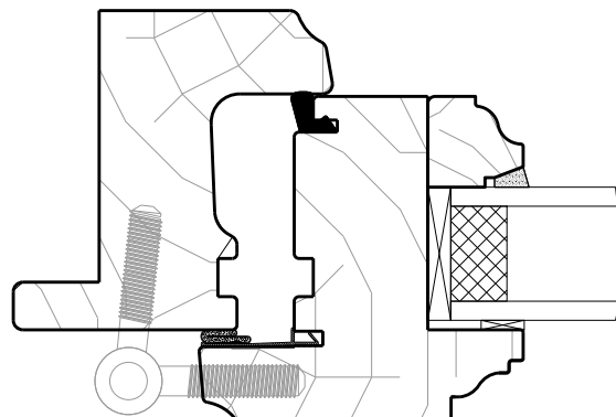
double joint sur ouvrant (portée extérieure et recouvrement intérieur)
