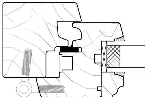
simple joint sur dormant
