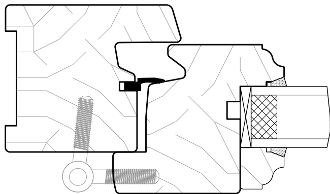
Simple joint sur dormant
