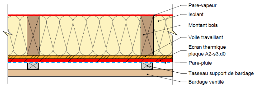
Mur - F1 - écran thermique plaque A2
