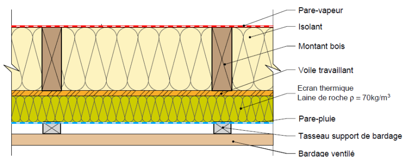
Mur - F2 - écran thermique laine de roche
