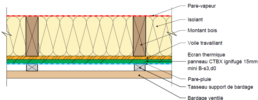
Mur - F3 - écran thermique CTBX ignifugé
